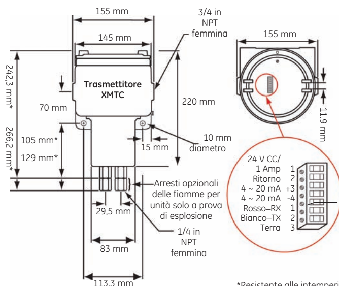
Dimensioni del trasmettitore della conducibilità termica XMTC
