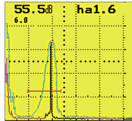
Live-Echo mit Hüllkurve (blau)
