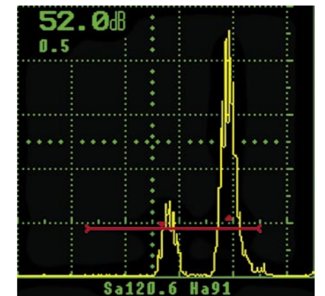
MESSPUNKT = Flanke: Schallweg am Schnittpunkt des ersten Echos mit der Blendenschwelle; Amplitude am höchsten Echo in der Blende
