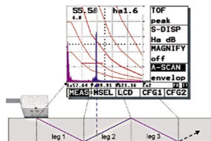
Farbwechsel bei der Schrägeinschallung
