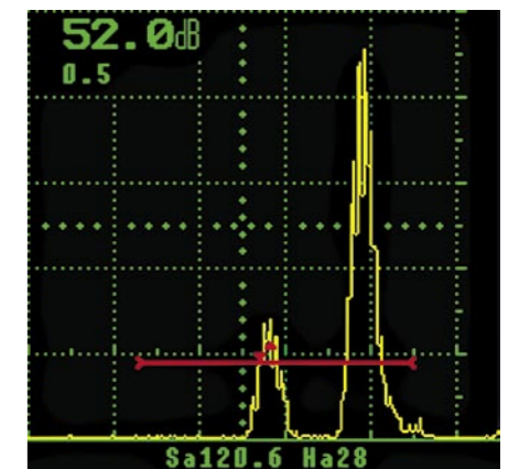
MESSPUNKT = JFlanke: Schallweg am Schnittpunkt des ersten Echos mit der Blendenschwelle; Amplitude ebenfalls am ersten Echo in der Blende
