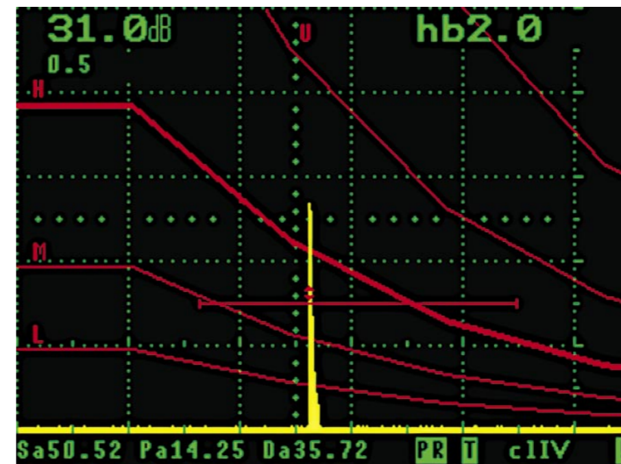
Zusätzlicher DAC nach japanischer Norm JIS Z3060-2002
