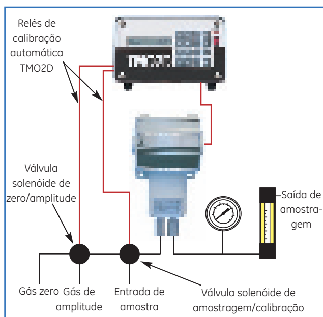
TMO2D com XMO2 e sistema de amostra
