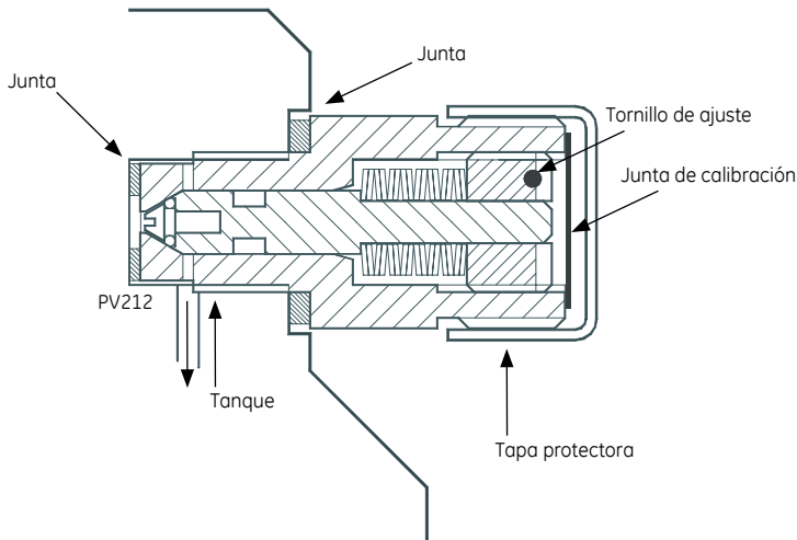
PRV212 Esquema
