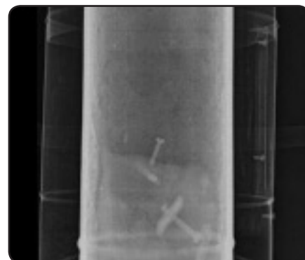
石油・ガスプラント配管の溶接部
