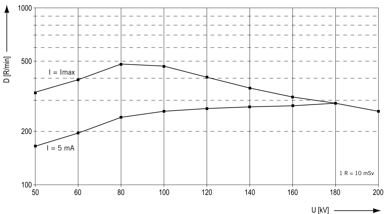
Dosisleistung (FDA 50 cm; 1 mm Be)
