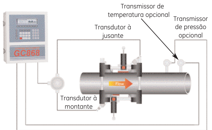
Configuração típica do medidor para vazão volumétrica padrão ou de massa de vapores
