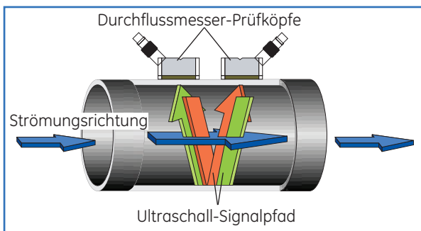
Laufzeit-Durchflussmessungstechnik
